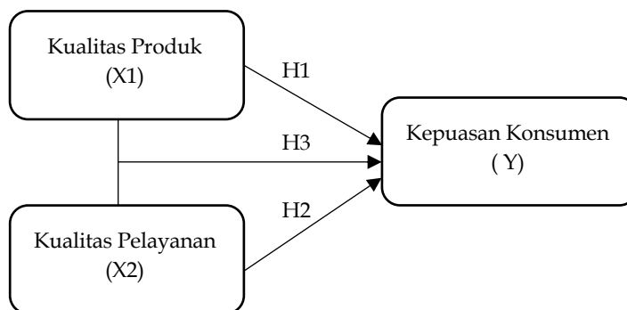
Gambar 1. Kerangka Penelitian
